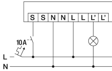
Standardbetrieb mit zusätzlicher Ansteuerung über Taster
